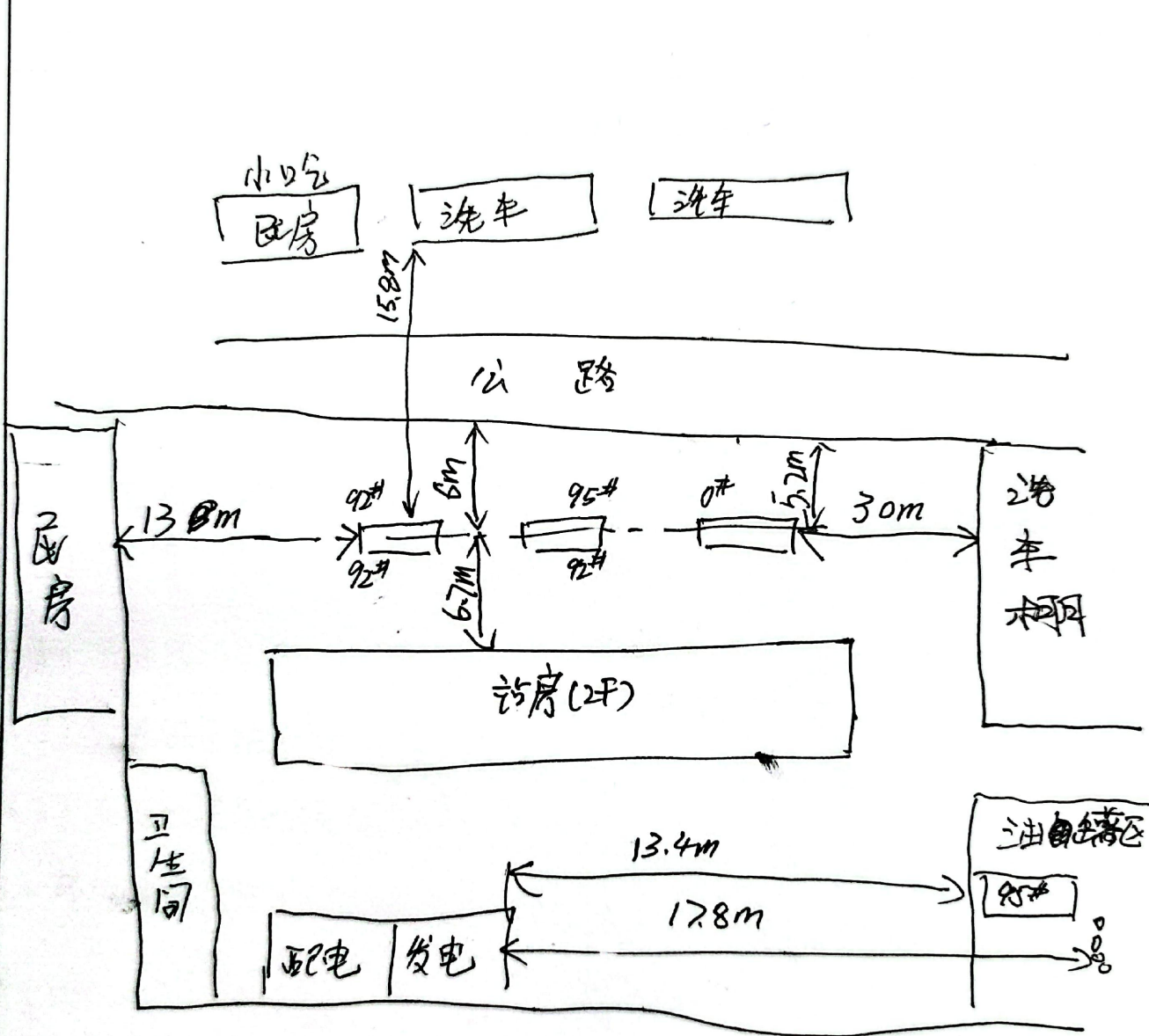
生产区域平面布置示意图
