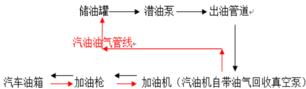
图 2-5 汽油加油流程框图
